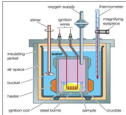
1 Spasi — { Gambar 3.2 Alat uji bom kalorimeter } 1 Spasi
